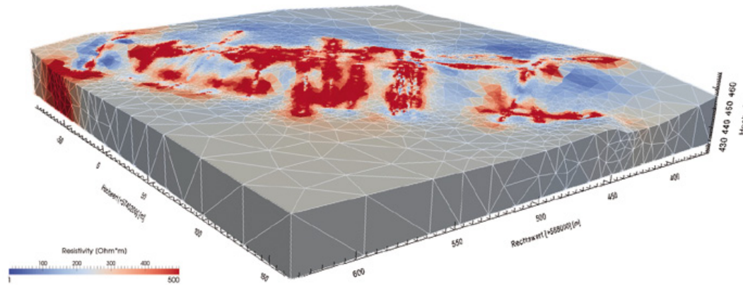
Geoelektrik-Modell einer Halde bei Clausthal/Zellerfeld, die u.a. Reststoffe, wie sogenannte Pochsande enthält. Durch ihre geringe elektrische Leitfähigkeit können die metallreichen Pochsande sichtbar gemacht werden.
