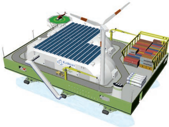
Konzept einer schiffgestützten Plattform zur Behandlung von Kunststoffabfällen
